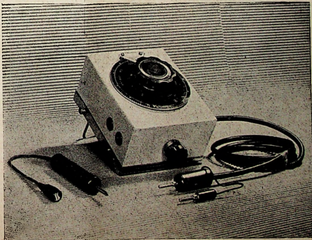
De Sonotron X Q-meter
